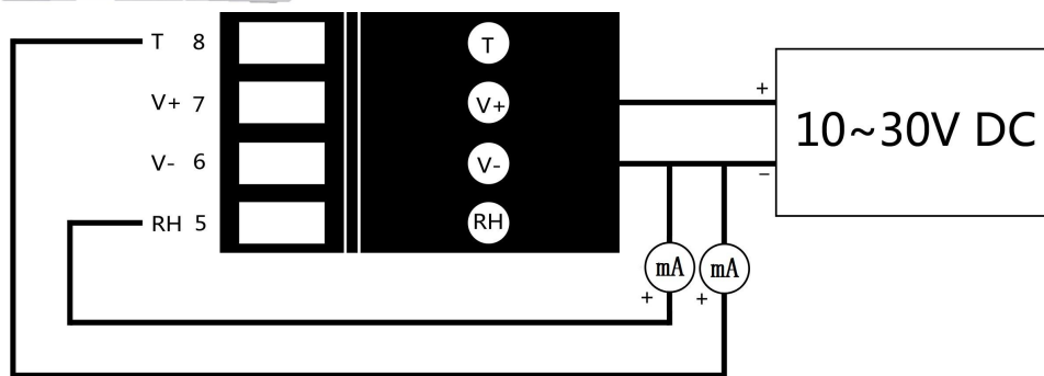
4~20mA 型电器连接图
