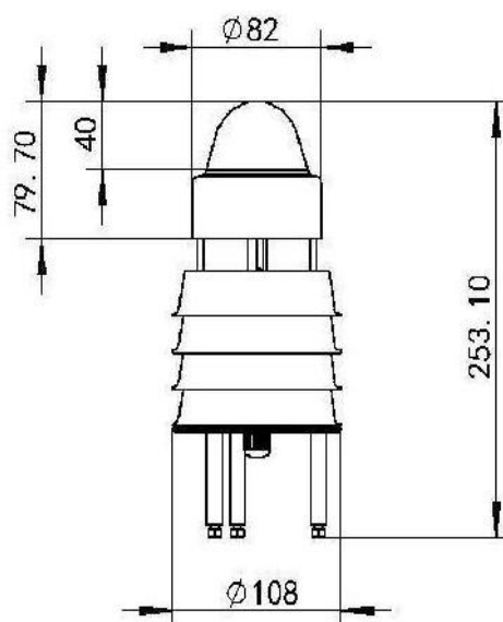
带光学雨量要素尺寸图 (单位: mm)
