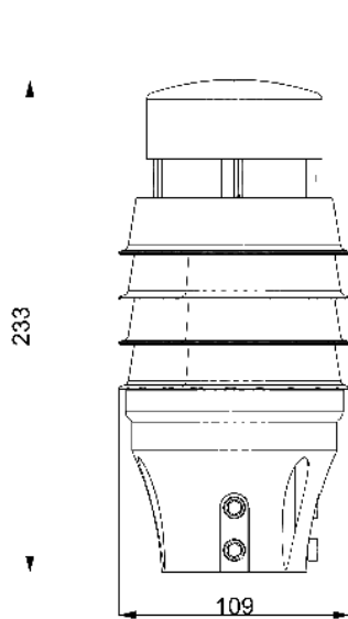
-3H 设备尺寸图 (单位: mm)
