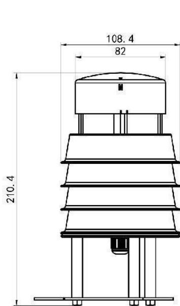
设备尺寸图 (单位: mm)
