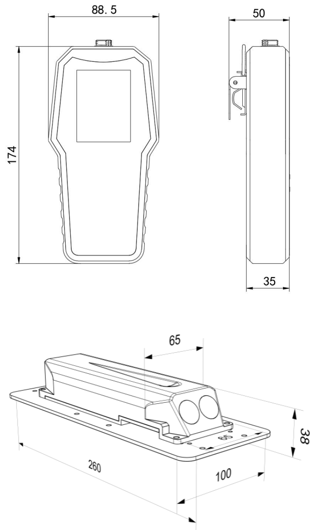
设备尺寸图（单位：mm）
