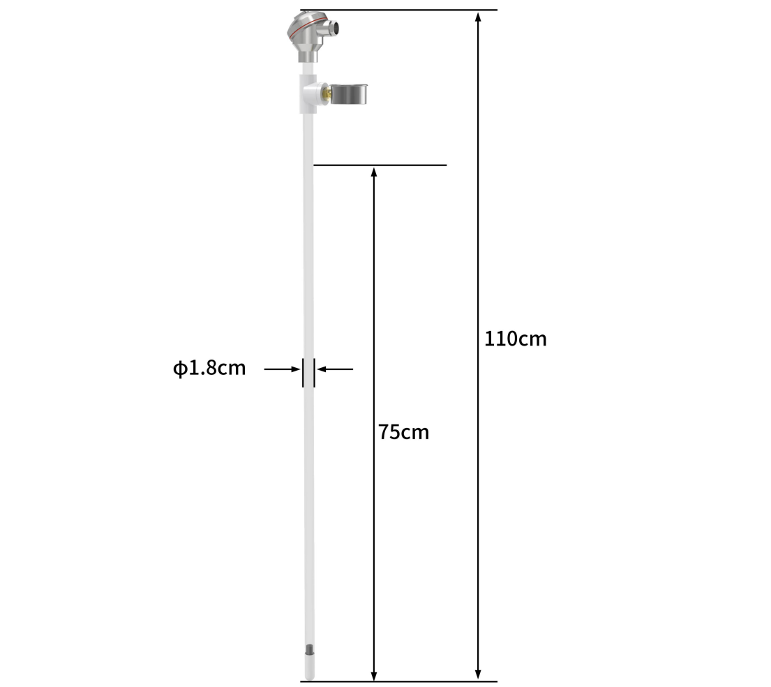
设备尺寸图（单位：mm）
