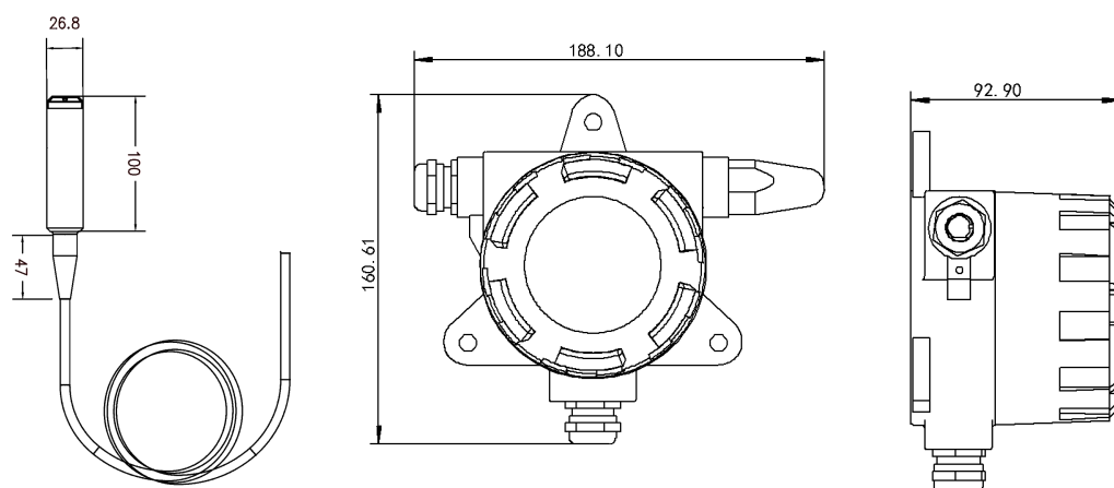
尺寸图 (单位: mm)
